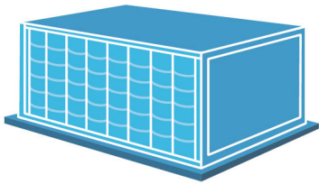
主艙集裝箱 - IATA 類型 2/2Q - IATA 前綴: AMA
